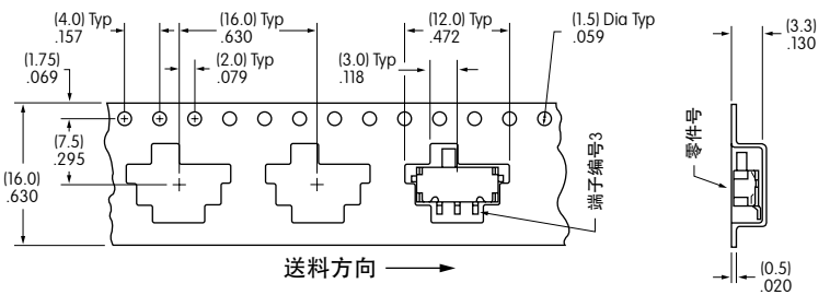
磁带尺寸
