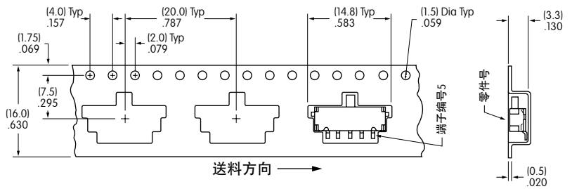
磁带尺寸
